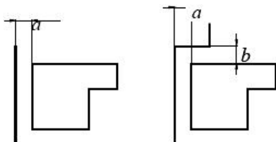
Рисунок 3 - Расположение монтажного зазора
