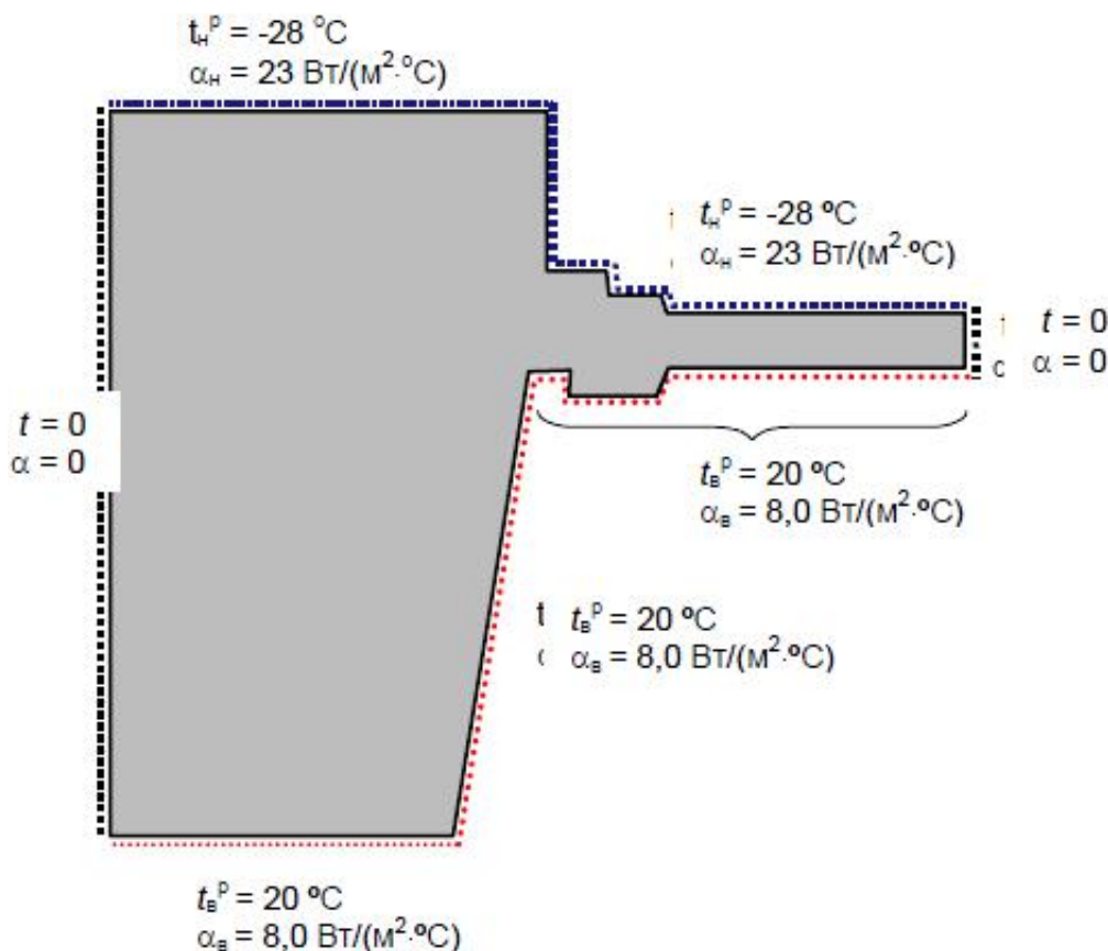
б) Схема заданий граничных условий
