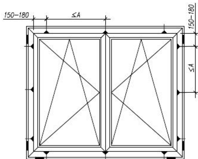
б) Оконный блок с безимпостным (шпательным) притвором
