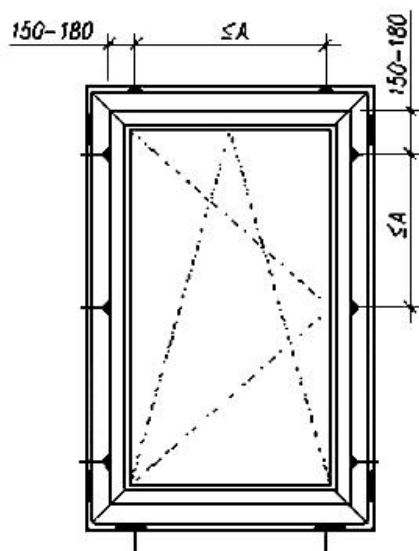
а) Оконный блок с поворотно - откидной системой открывания створки
